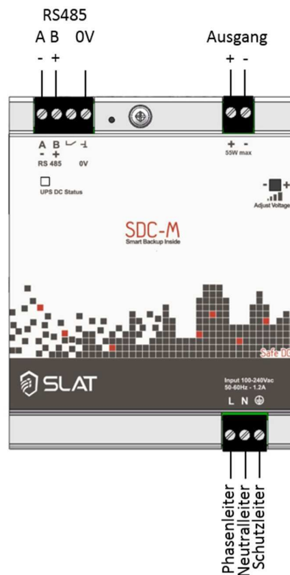
Abb. 6.2: Verkabelung
