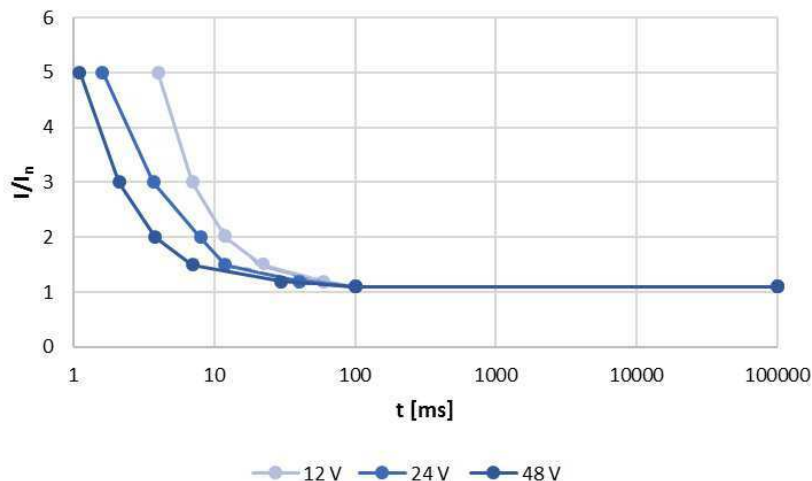
Abb. 10.4: Überlast-Kennlinie
