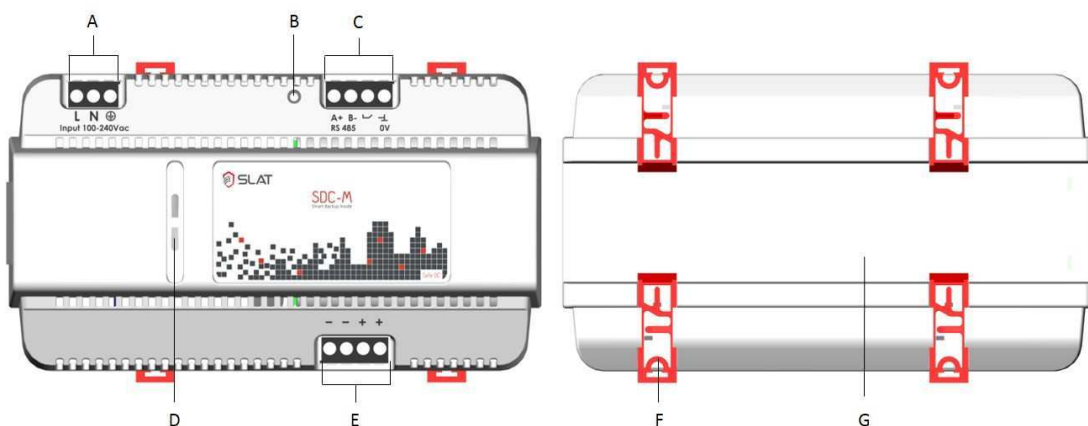
Abb. 4.2: Produktansicht
