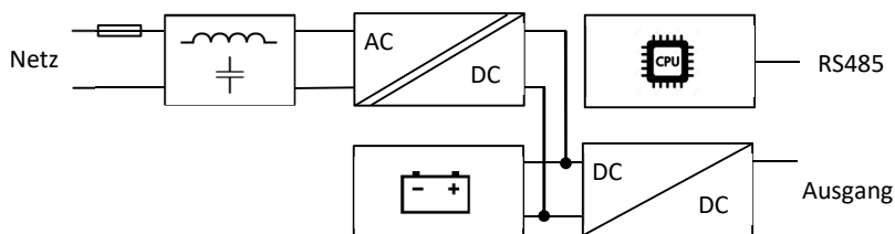
Abb. 4.1: Prinzipschema
