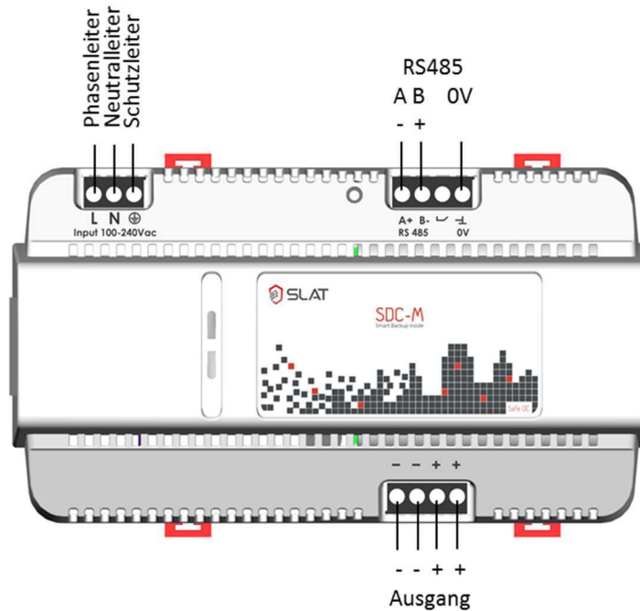
Abb. 6.3: Verkabelung
