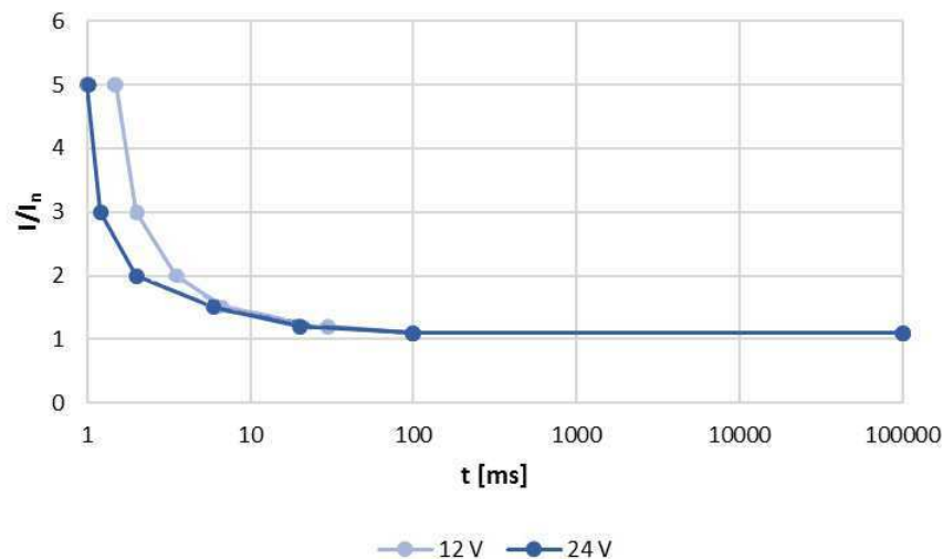
Abb. 10.4: Überlast-Kennlinie
