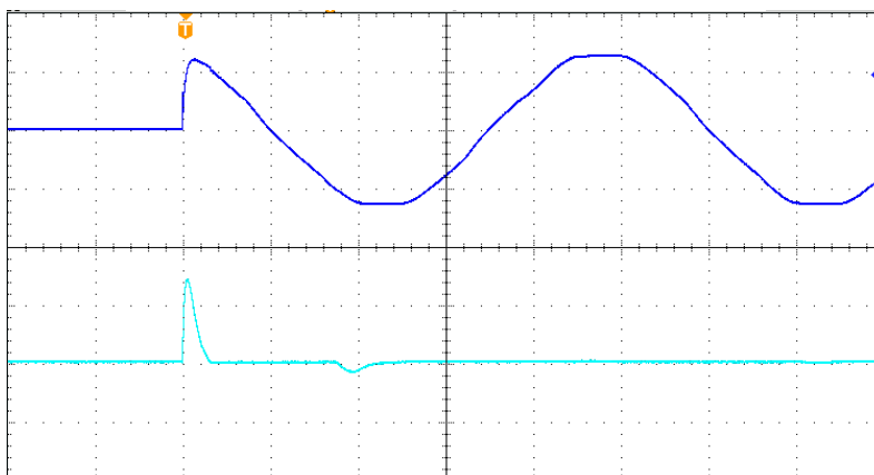
Abb. 10.1: Oszillogramm - Einschaltstrom
