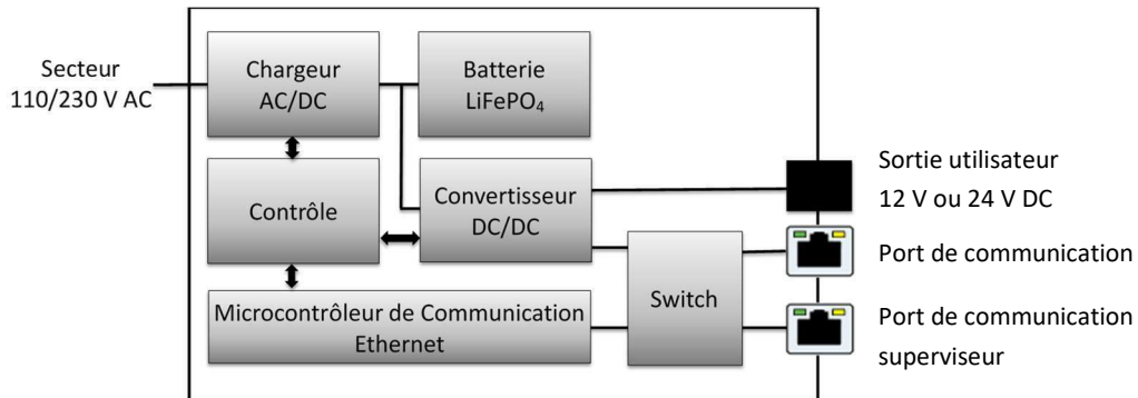
Figure 6.1: Schéma de principe
