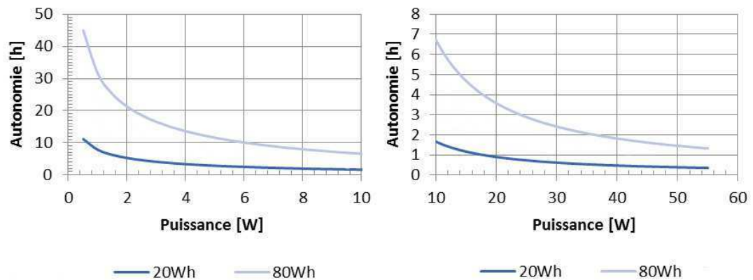
Figure 7.2: Courbes d'autonomie
