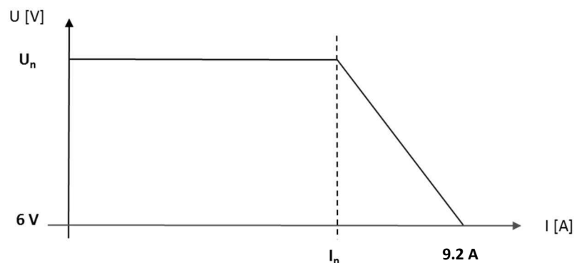
Figure 12.3: Tension de sortie vs Courant d'utilisation
