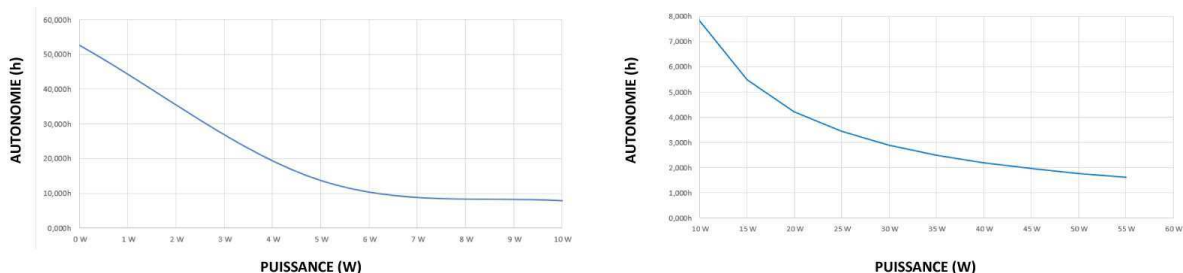
Figure 7.3: Courbes d'autonomie Backup G à 20°C
