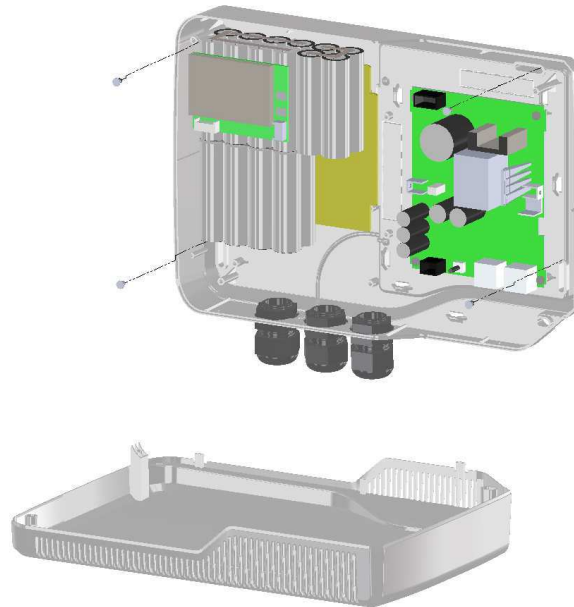
Figure 8.4: Fixation avec vis
