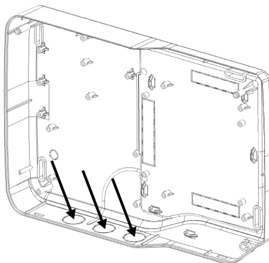
Figure 8.1: Passage de câbles en bas
