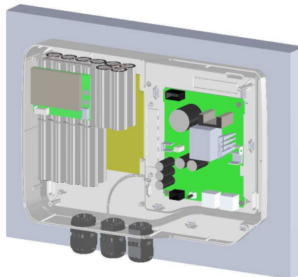
Figure 8.5: Montage au mur
