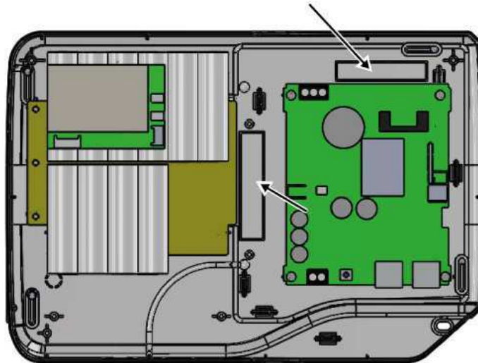
Figure 8.3: Passage de câbles par l'arrière
