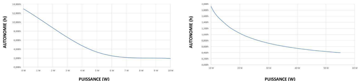
Figure 7.2: Courbes d'autonomie Backup D à 20°C
