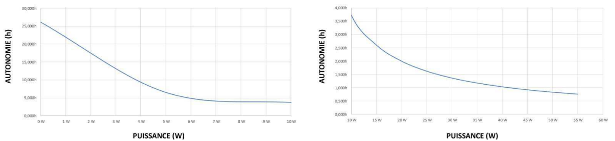
Figure 7.3: Courbes d'autonomie E à 20°C
