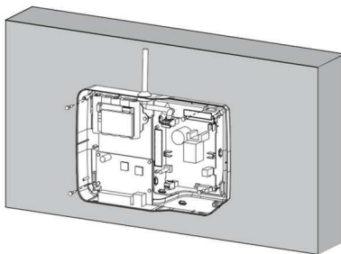
Figure 8.2: Montage au mur
