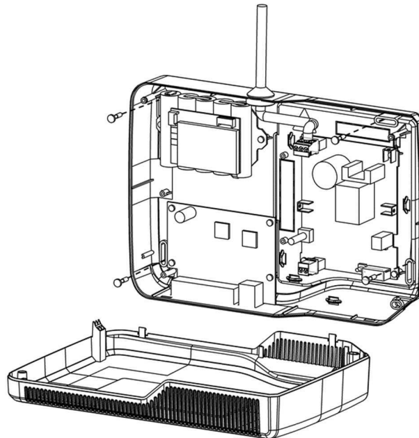
Figure 8.1: Fixation avec vis
