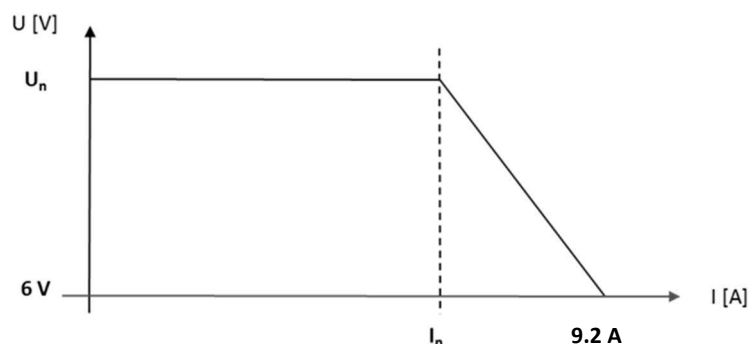
Figure 12.2: Tension de sortie vs Courant d'utilisation
