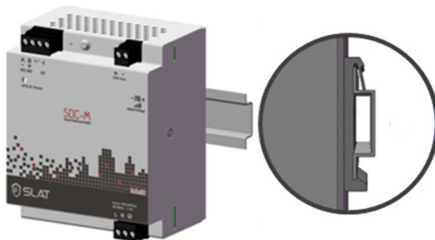
Abb. 6.1: Anbringung an DIN-Schiene
