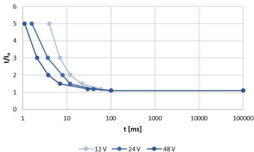
Abb. 10.4: Überlast-Kennlinie
