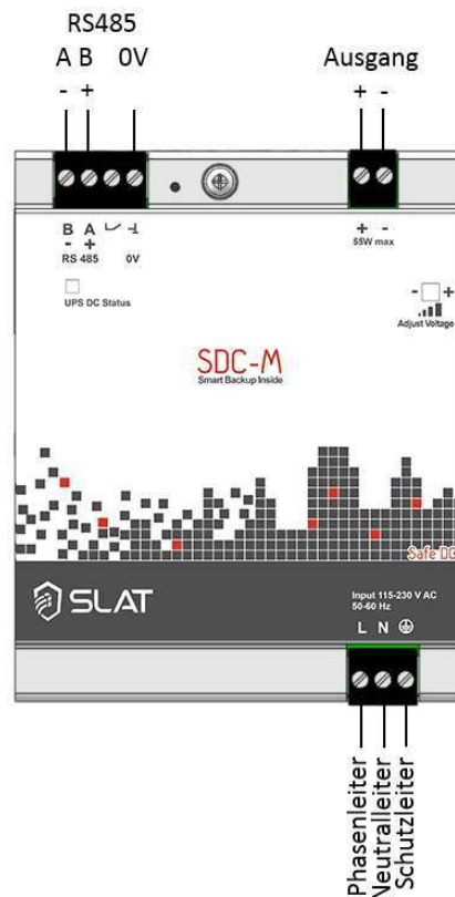
Abb. 6.2: Verkabelung
