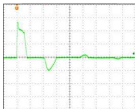
Figure 12-1 - Oscillogramme - courant de démarrage
