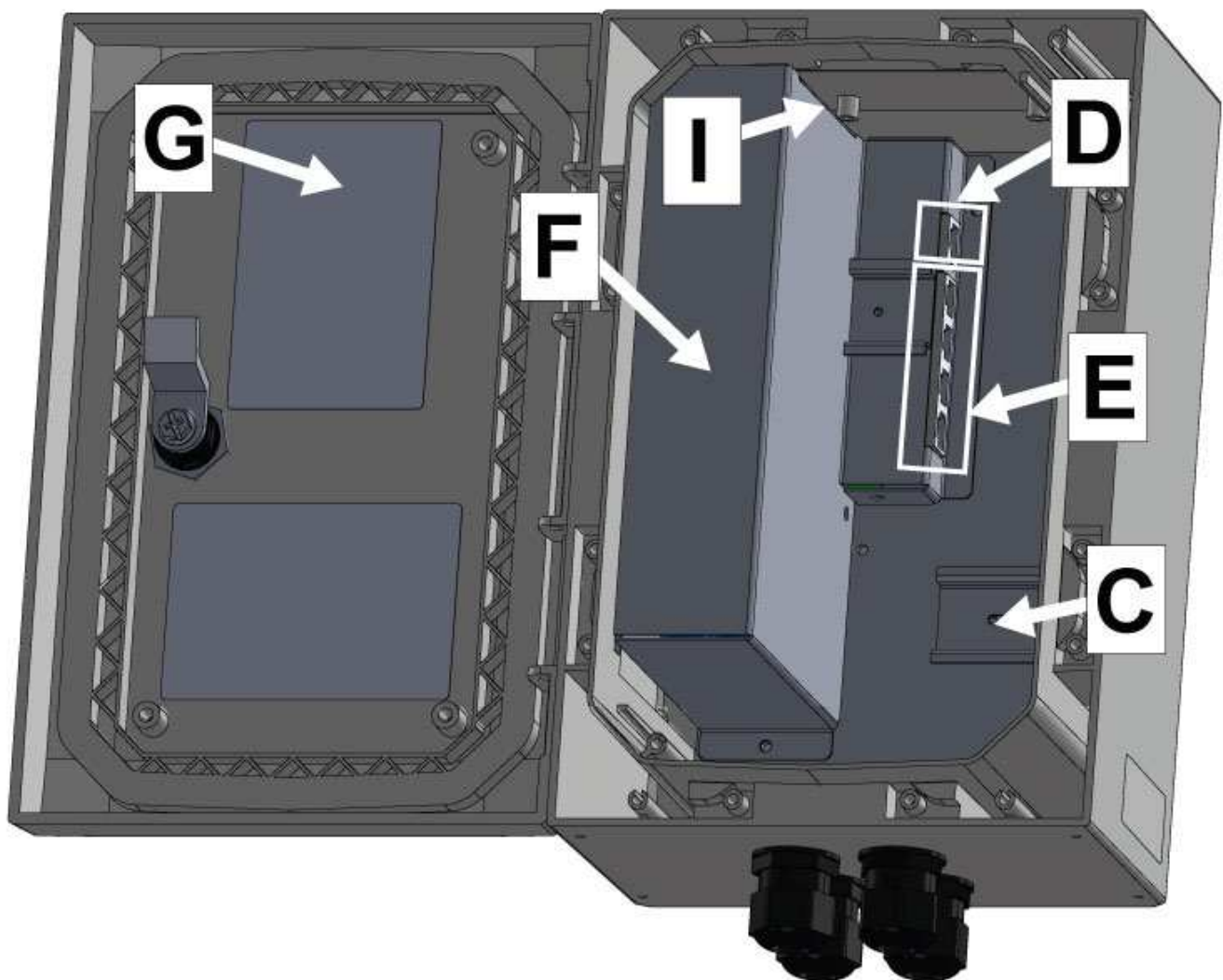
Vue de l'intérieur (modèle SYNAPS-POE 3E P4)
