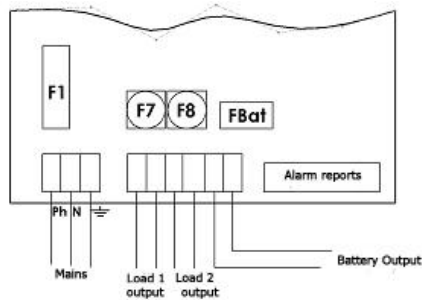
50-75W wiring
