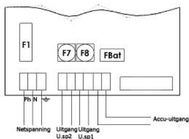
Kabels 50-75W
