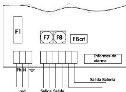
Cableado 50-75 W
