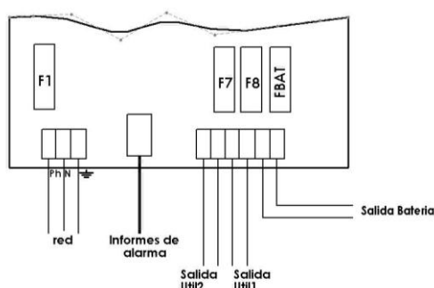
Cableado 100-600 W
