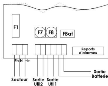
Câblage 50-75W
