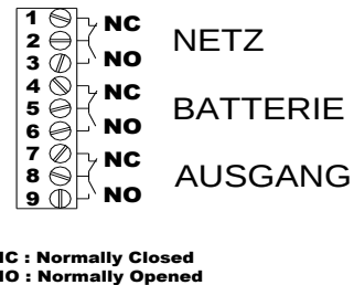
Verkabelung Fernmeldung
