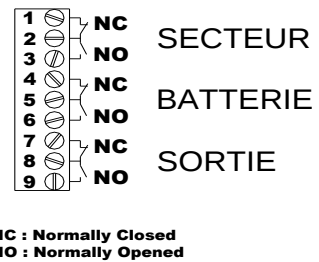
Câblage reports d'alarmes
