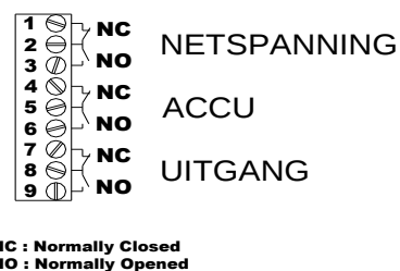
Kabels alarmoverdracht
