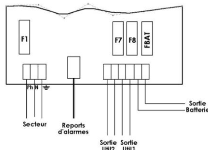
Câblage 100-600W
