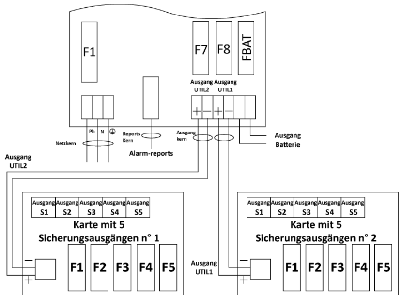
Abb.4 Verkabelung mit 2 Karten mit 5 Sicherungsausgängen (optional für Gehäuse C85)
